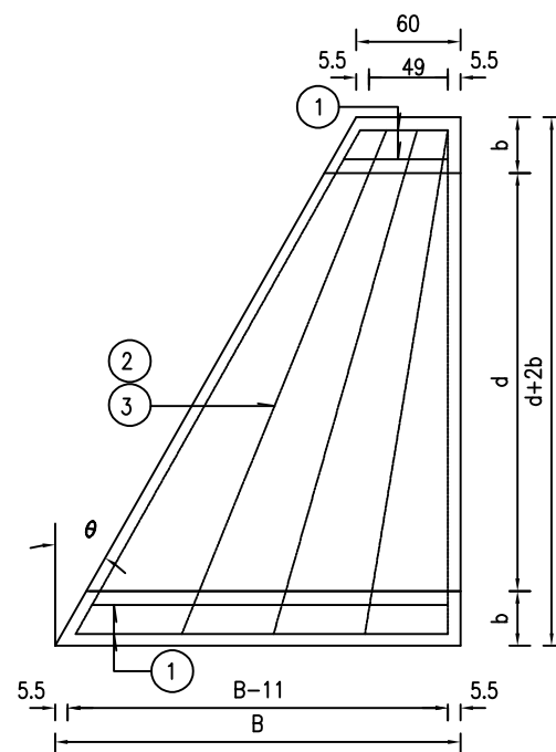
纵 断 面 1:30
