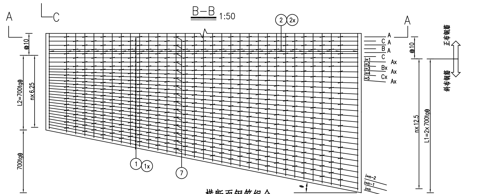
横断面钢筋组合
