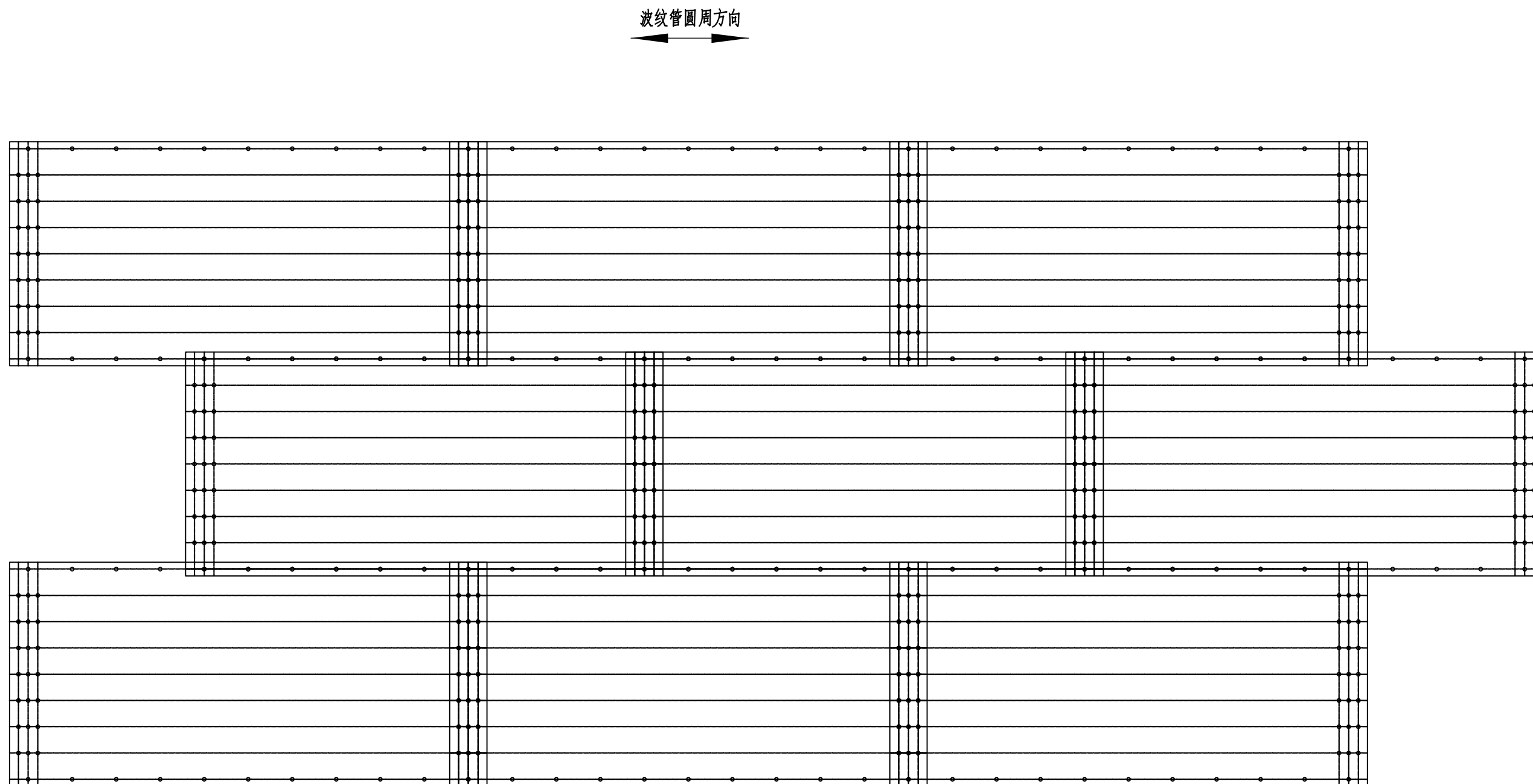
分片拼装钢制波纹管周向连接示意图
