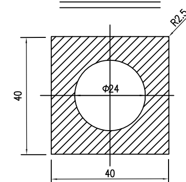
凹垫圈平面图
