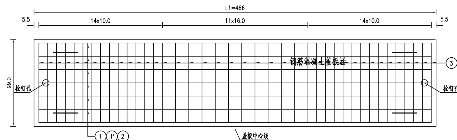
盖板平面
