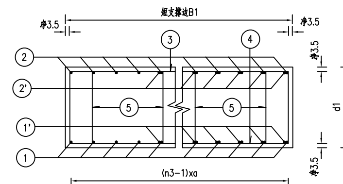
A - A 1:25
