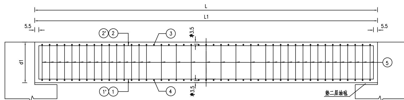
盖板断面 1:25
