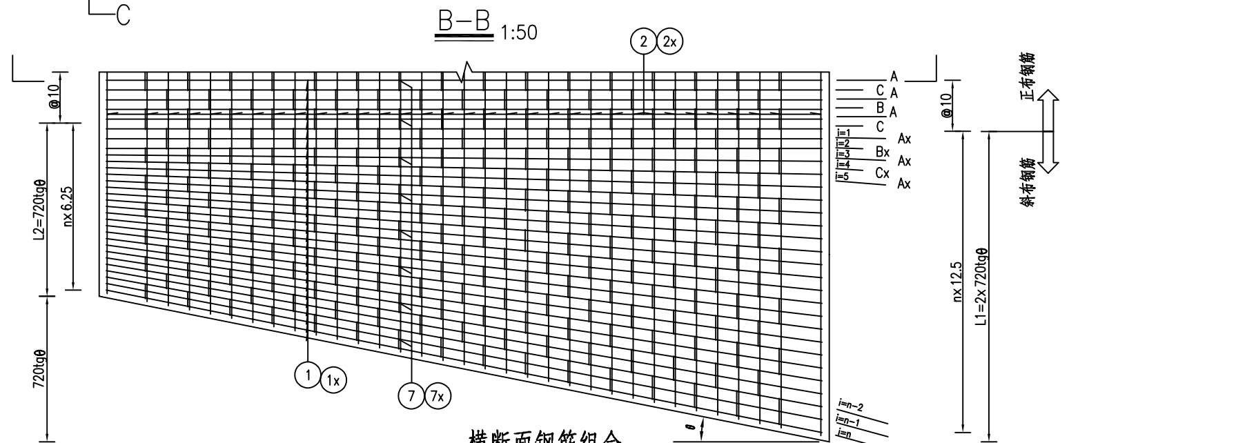
横断面钢筋组合
