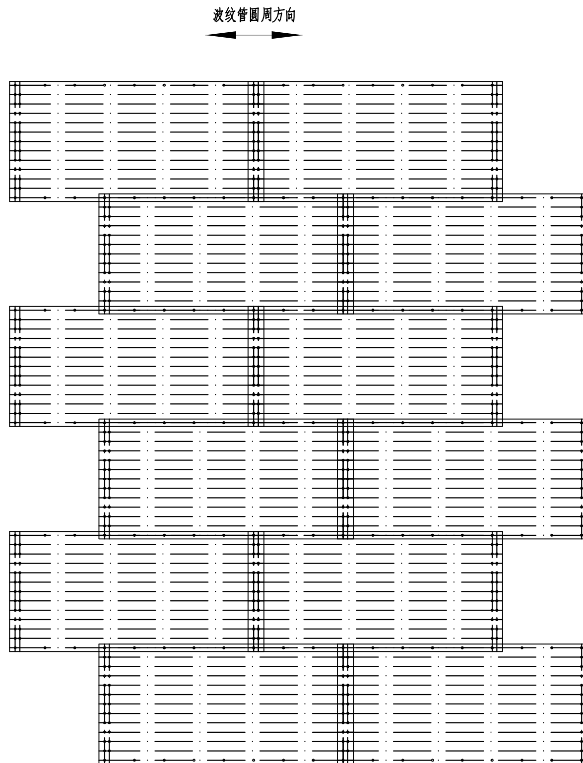
分片拼装钢制波纹管周向连接示意图
