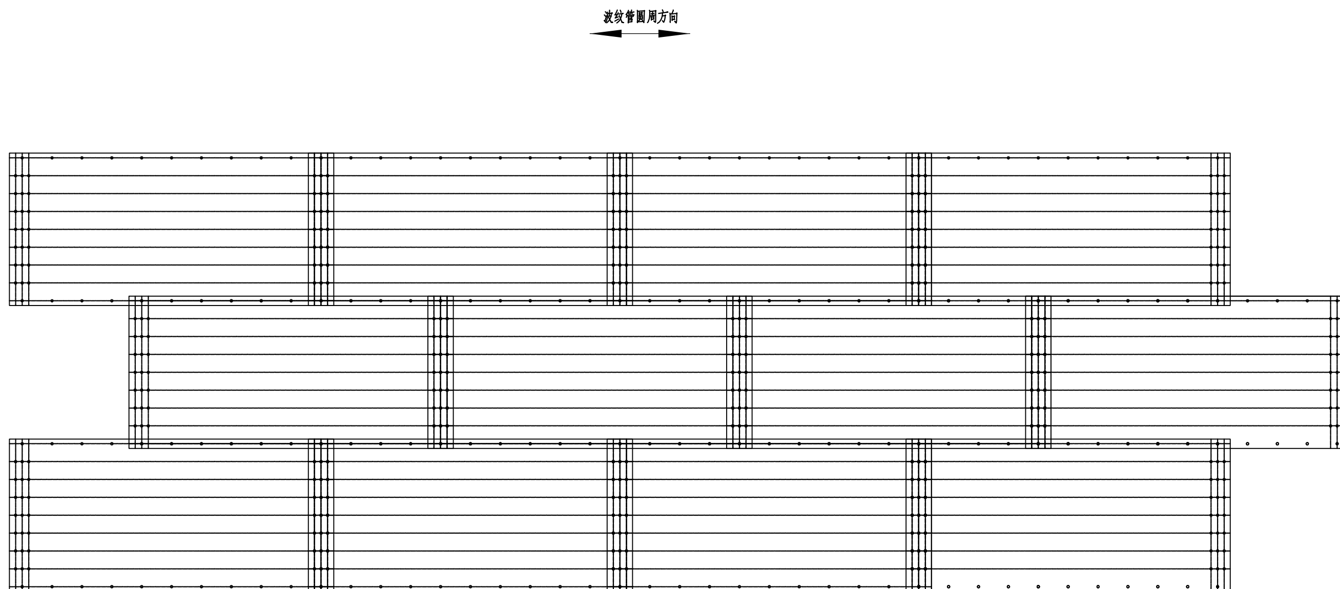
分片拼装钢制波纹管周向连接示意图
