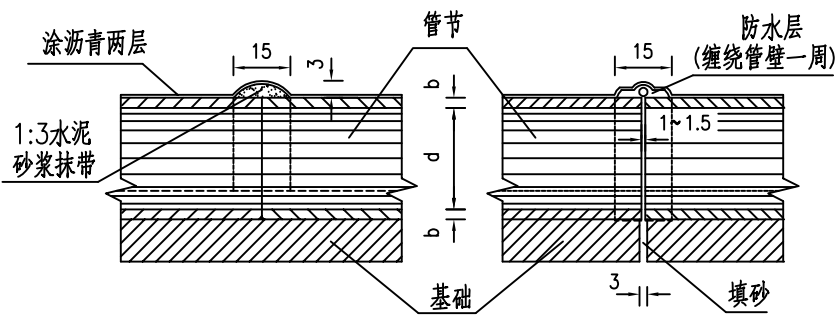
管节接头
