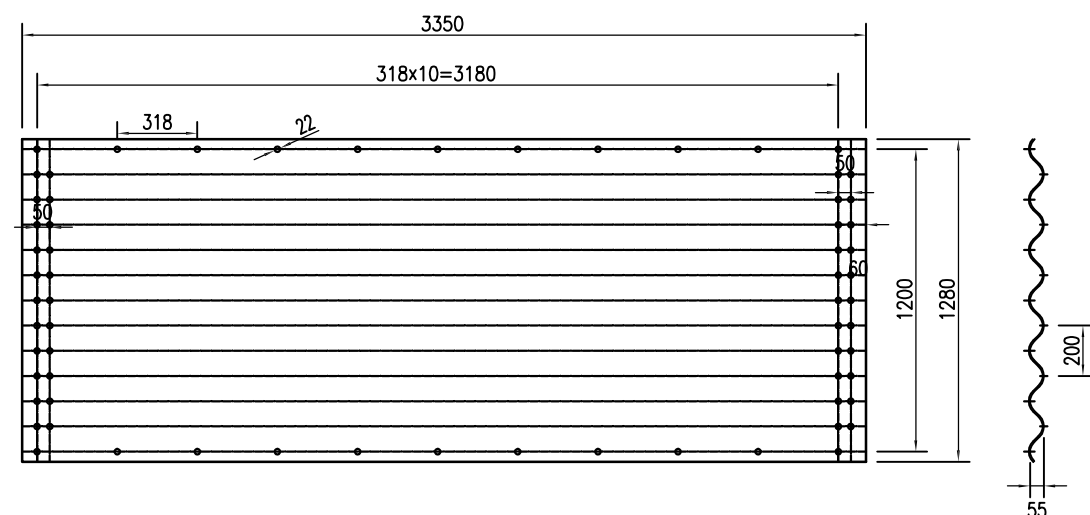
波纹板片周向展开平面图
