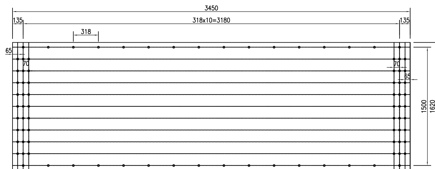
波纹板片周向展开平面图
