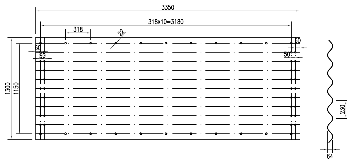
波纹板片周向展开平面图
