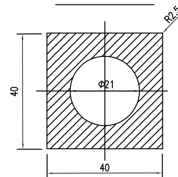
凹垫圈平面图
