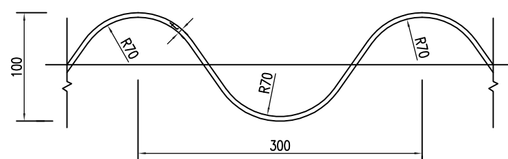
波纹板波形大样图
