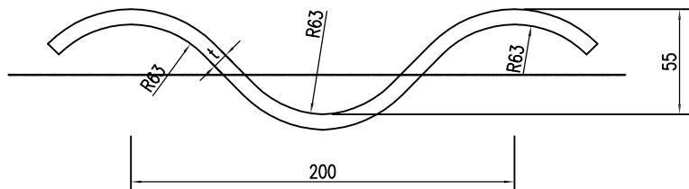
波纹板波形大样图
