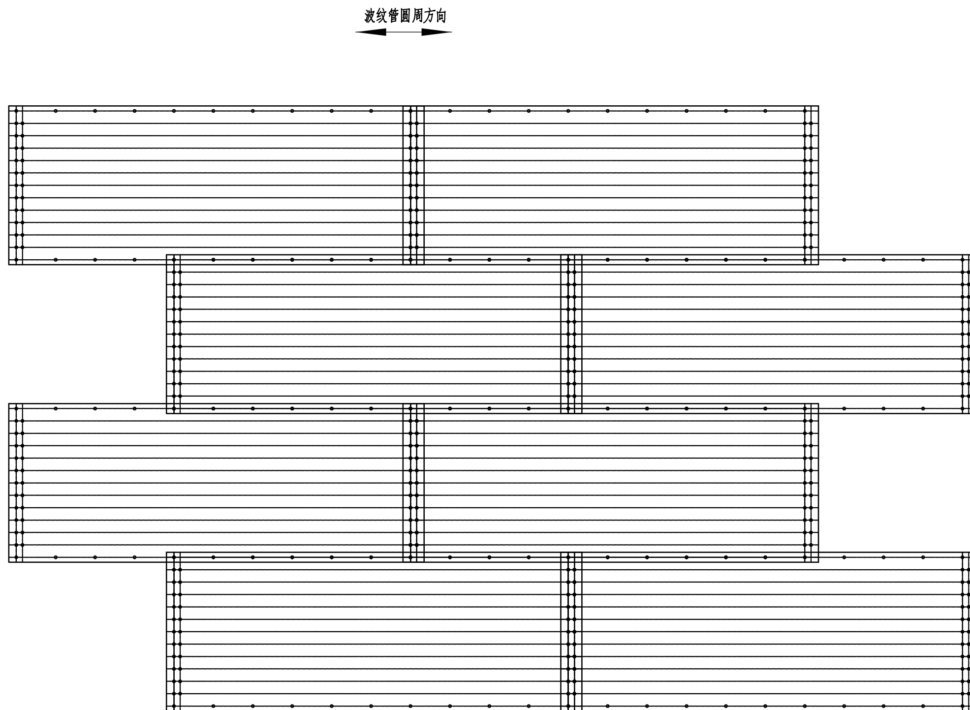
分片拼装钢制波纹管周向连接示意图
