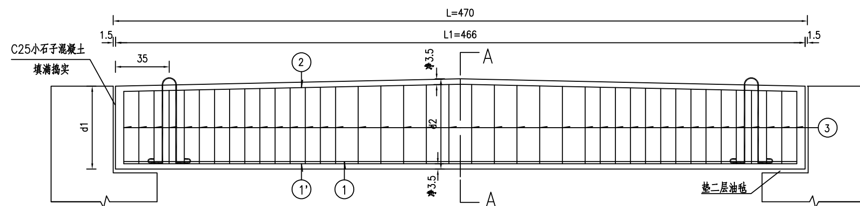
盖板断面
