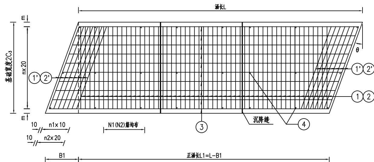
整体式基础钢筋平面布置图
