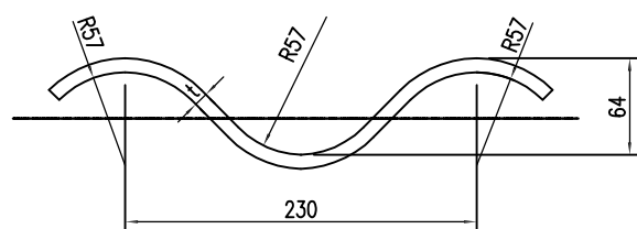
波纹板波形大样图
