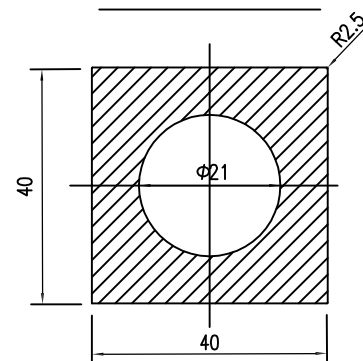
凸垫圈平面图
