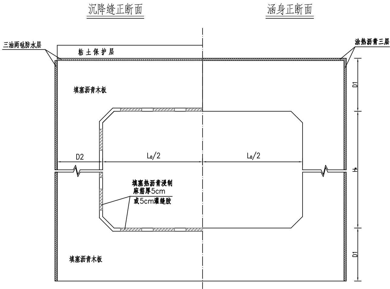
沉降缝、防水构造立面图
