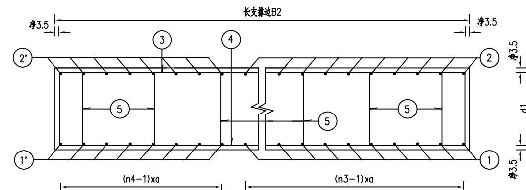
B - B 1:25
