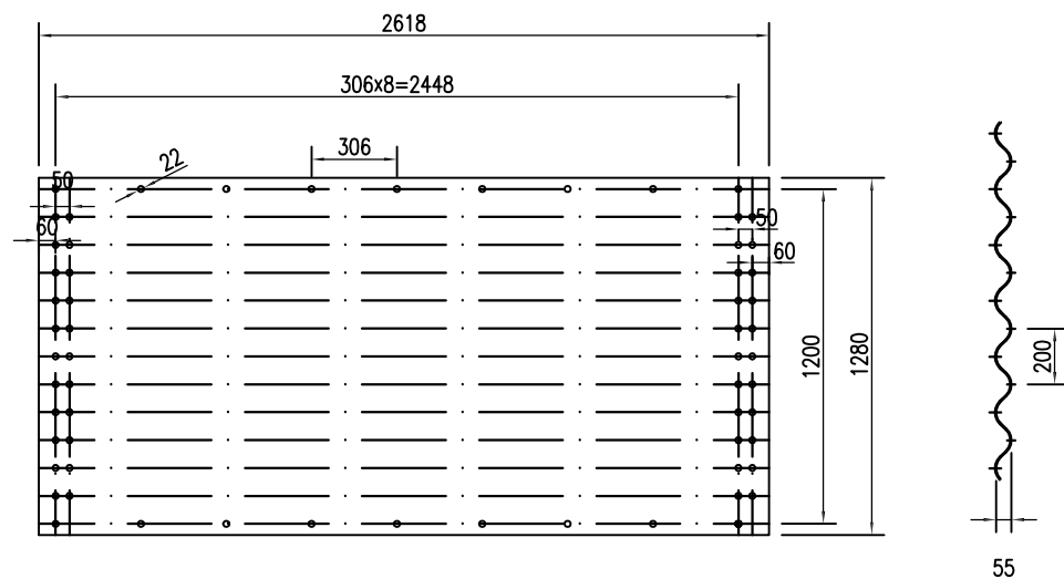
波纹板片周向展开平面图
