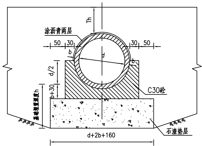
单孔涵洞管基构造
